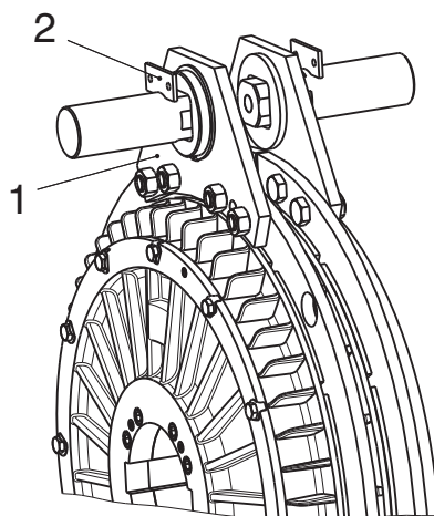
Obr. 5: Zavěšení dvoubodové
