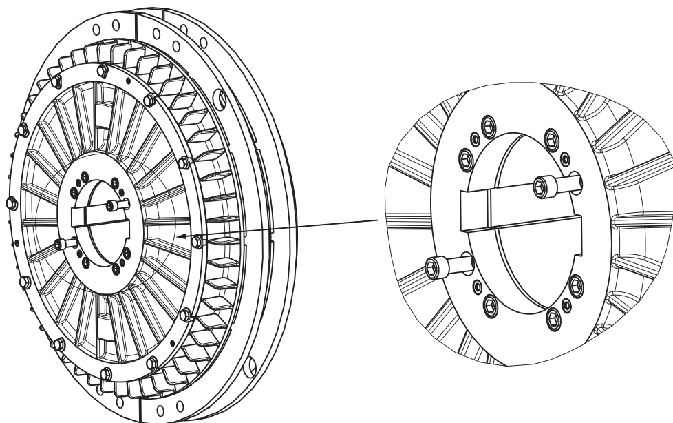
Obr. 13: Šrouby spojující válec-nosník
