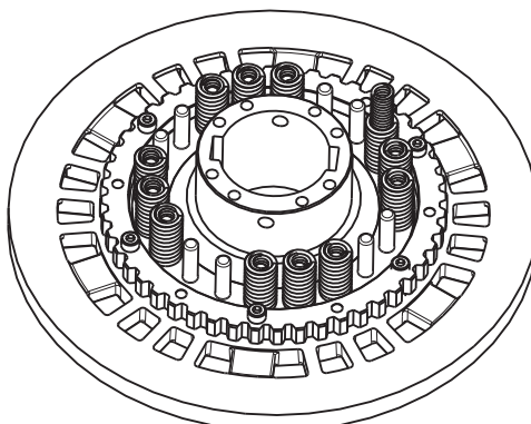
Obr. 10: Rozmístění přitlačných pružin
