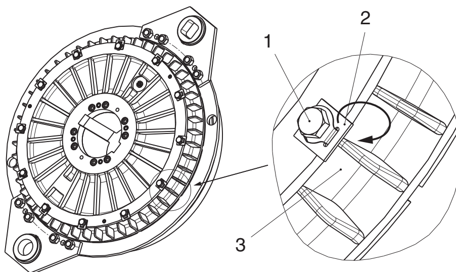
Obr. 8: Vyrovnání opotřebení
