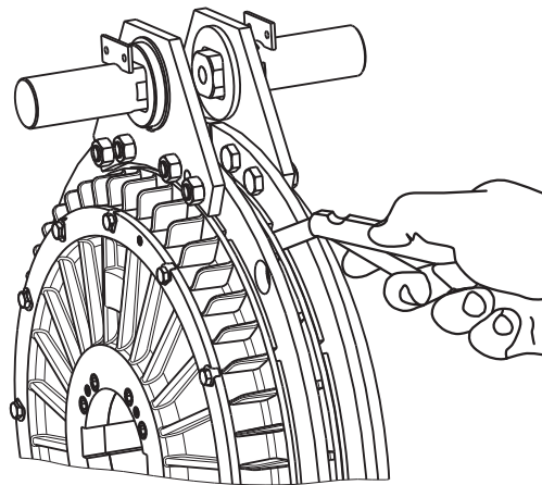
Obr. 6: Kontrola opotřebení
