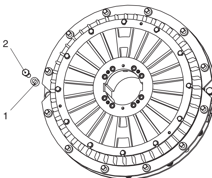
Obr. 4: Dvanáctibodové upevnění (verze s třecími špalíky)
