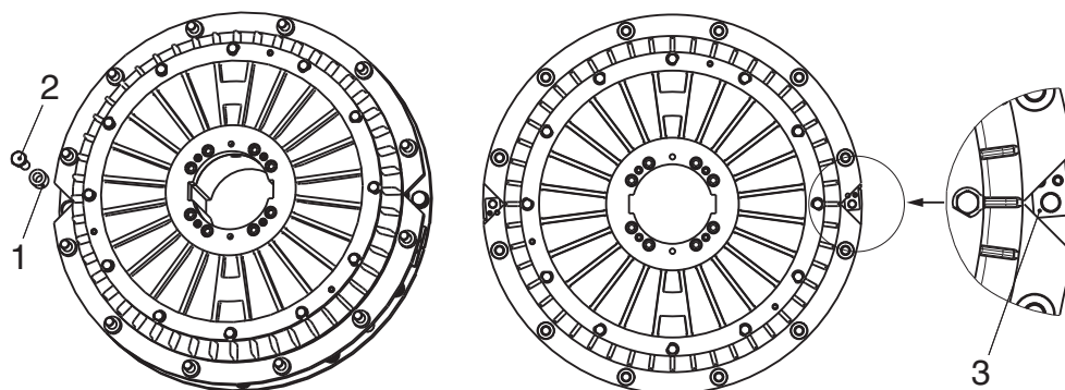
Obr. 2: Dvanáctibodové zavěšení
