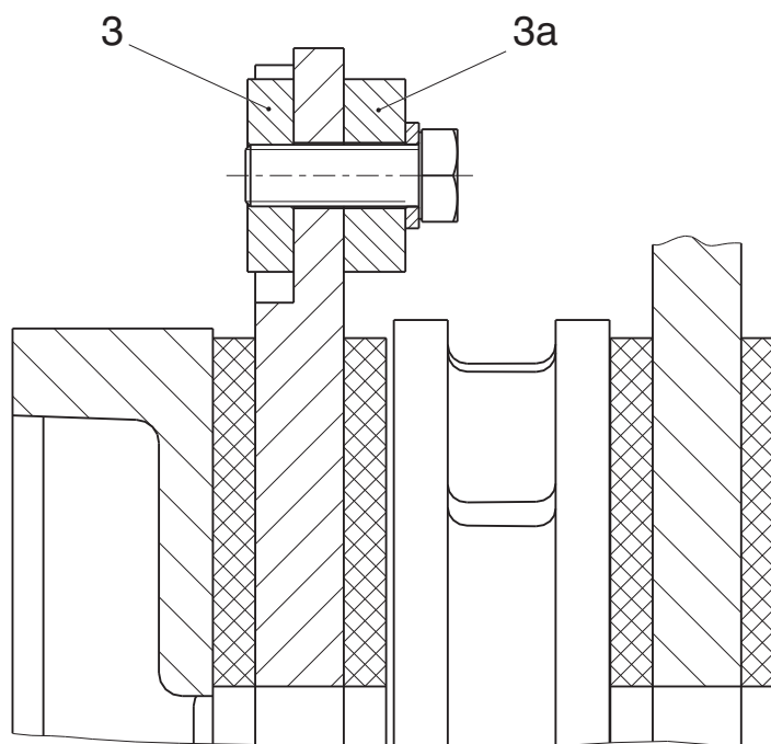
Obr. 3: Dvanáctibodově zavěšení s dvojitým překrývaným spojením od velikosti 90
